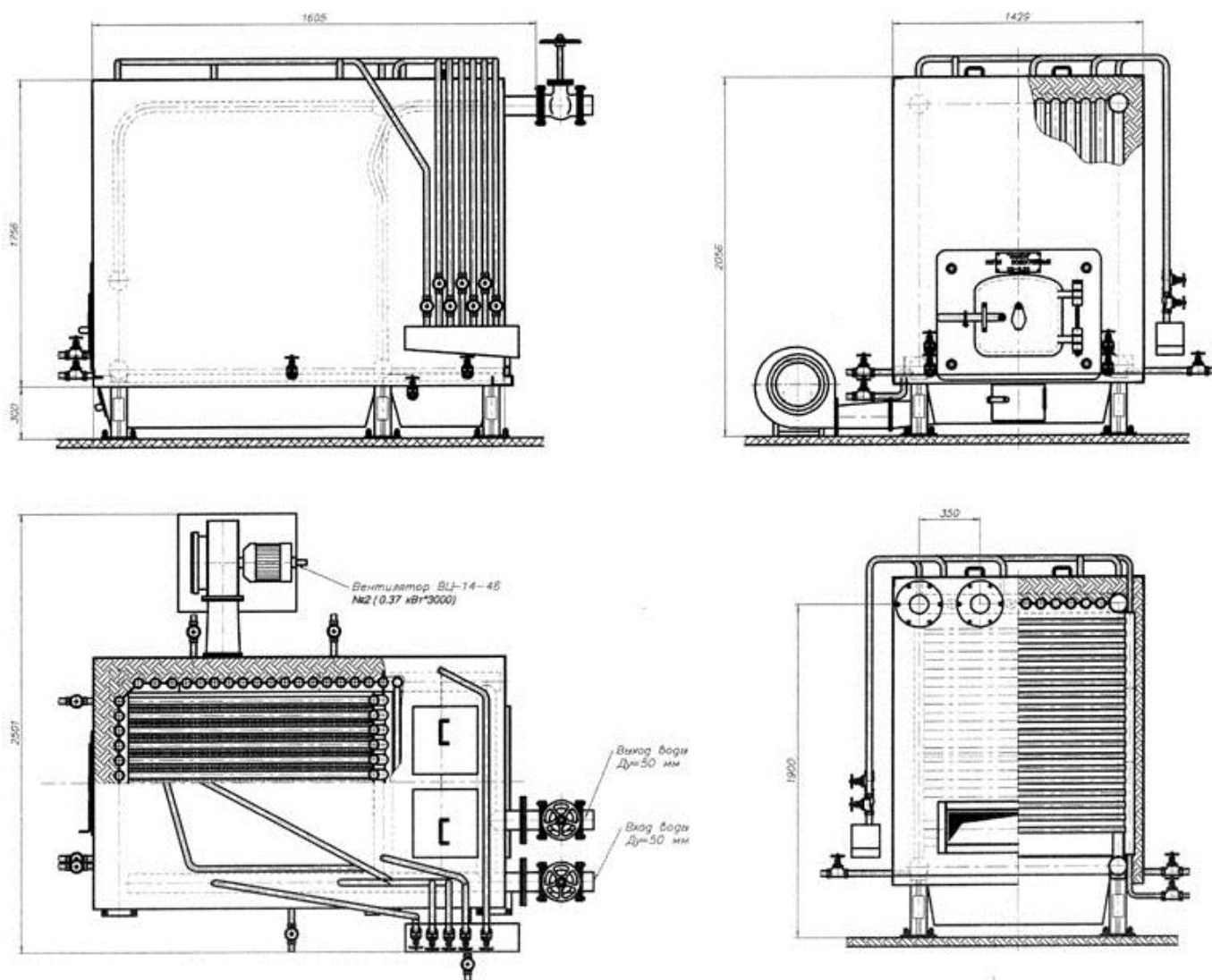
Рисунок 2.1 – Устройство и габариты компоновки котла КВр-0.3
