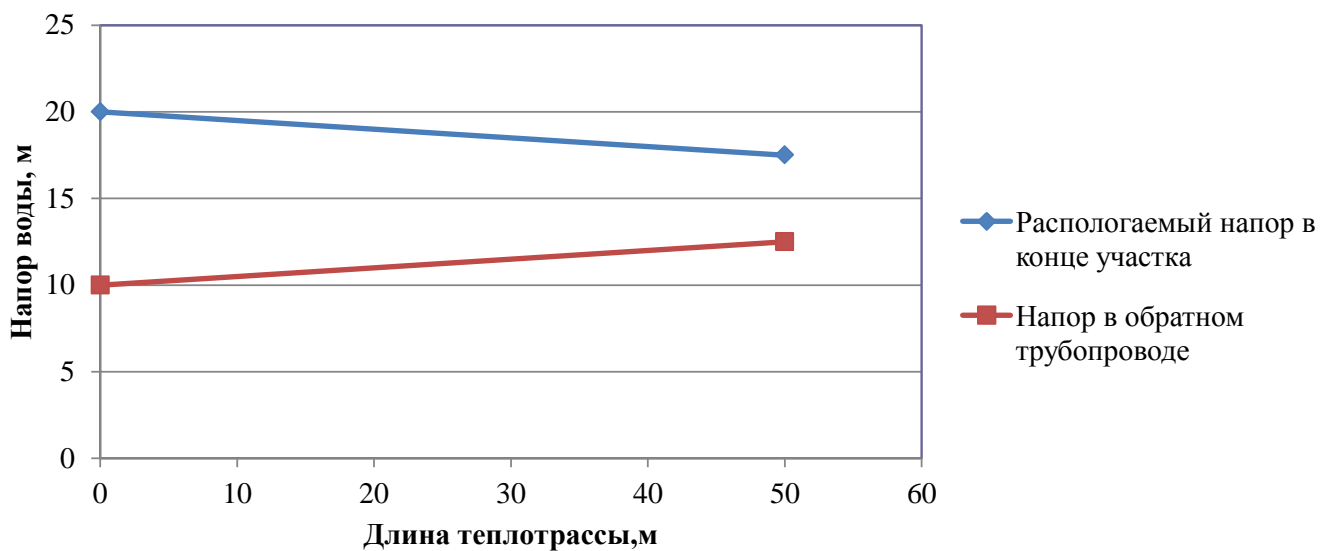
Рисунок 2.8 – Пьезометрический график тепловой сети ЦРБ
