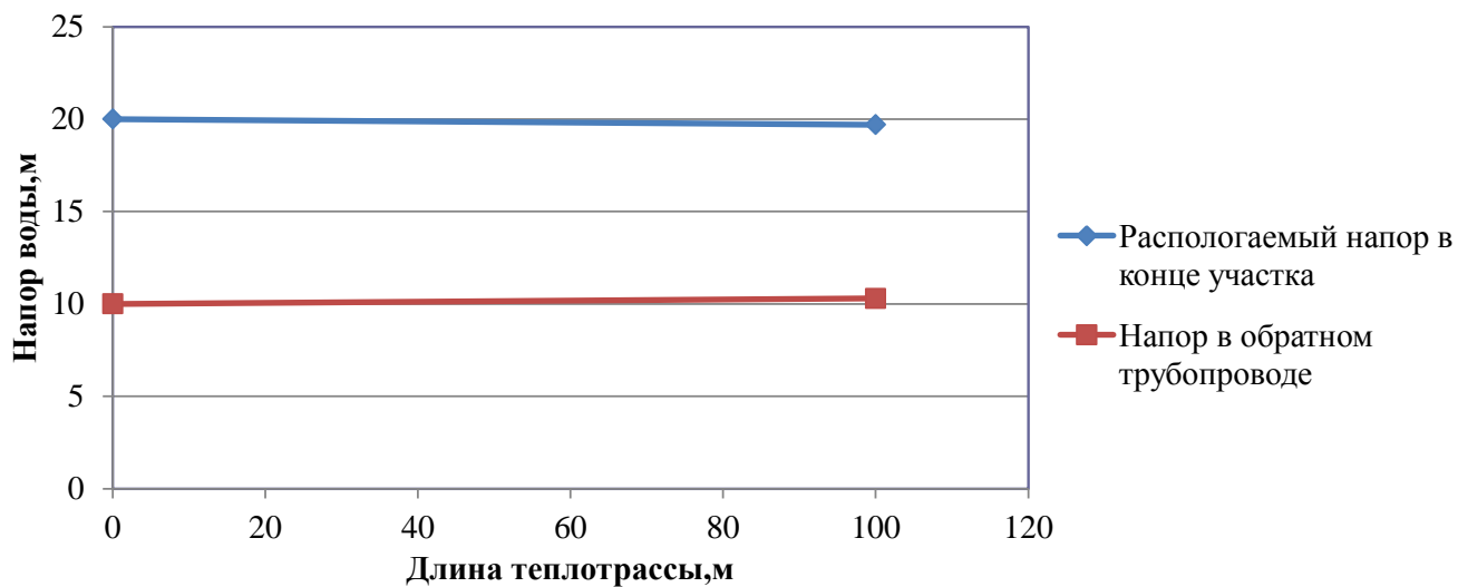
Рисунок 2.5 – Пьезометрические графики тепловой сети с. Целинное: а) участок котельная №1; б) котельная – школа; в) котельная – ЦРБ
