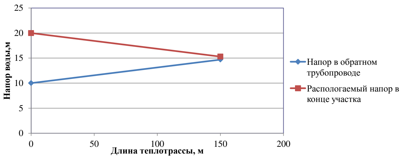
Рисунок 2.7 – Пьезометрический график тепловой сети от котельной №2
