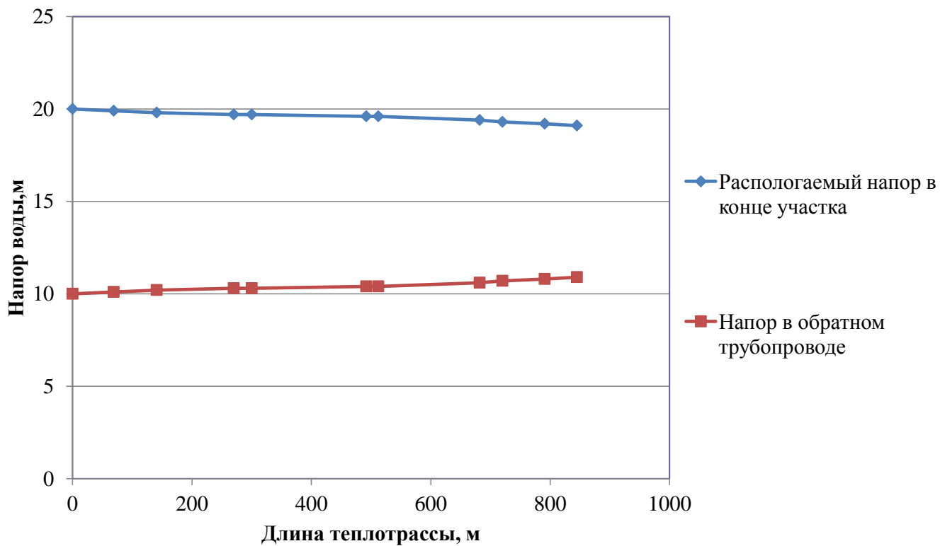
Рисунок 2.6 – Пьезометрический график тепловой сети от котельной №1
