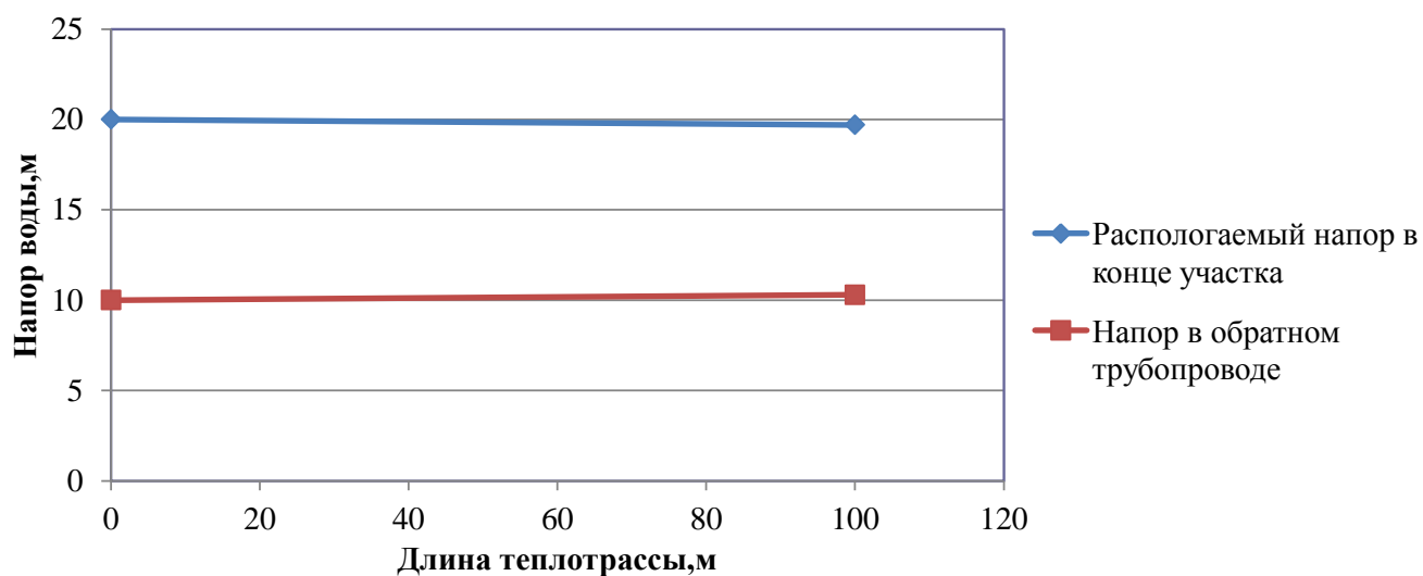
Рисунок 2.9 – Пьезометрический график тепловой сети детского сада и колледжа
