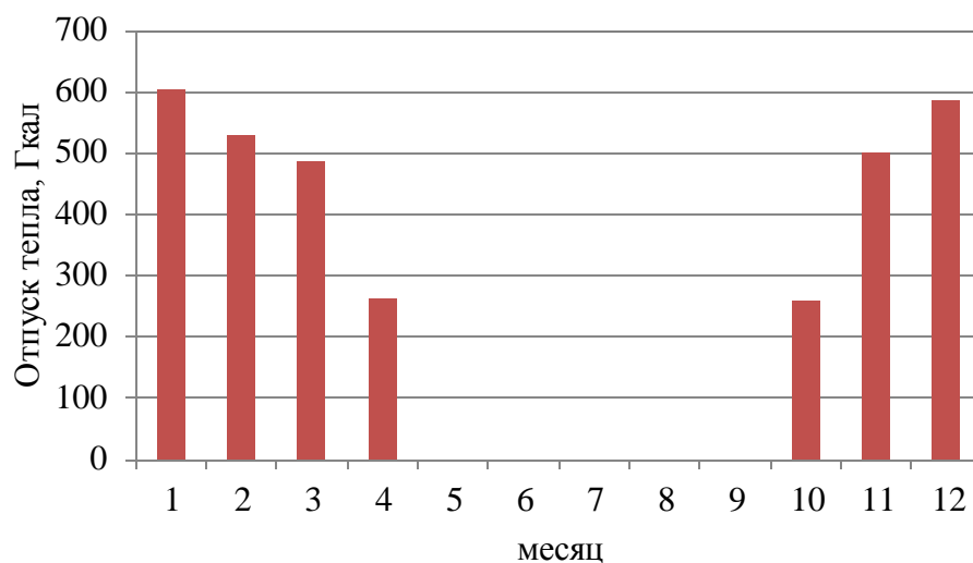
Рисунок 1.3 – Оптимальный температурный график отпуски тепловой энергии для муниципальной котельной с. Целинное
