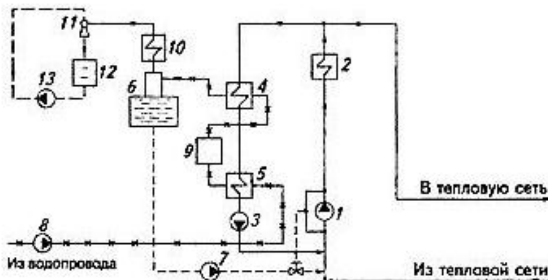
Рисунок 2.2 – Принципиальная тепловая схема котельной с водогрейными котлами: 1 - сетевой насос; 2 - водогрейный котел; 3 - рециркуляционный насос; 4 - подогреватель подпиточной воды; 5 - подогреватель водопроводной воды; 6 - вакуумный деаэратор; 7 - подпиточный насос и регулятор подпитки; 8 - насос водопроводной воды; 9 - оборудование химводоподготовки; 10 - охладитель выпара; 11 - вакуумный водоструйный эжектор; 12 – бак газоотделитель эжектора; 13 - эжекторный насос
