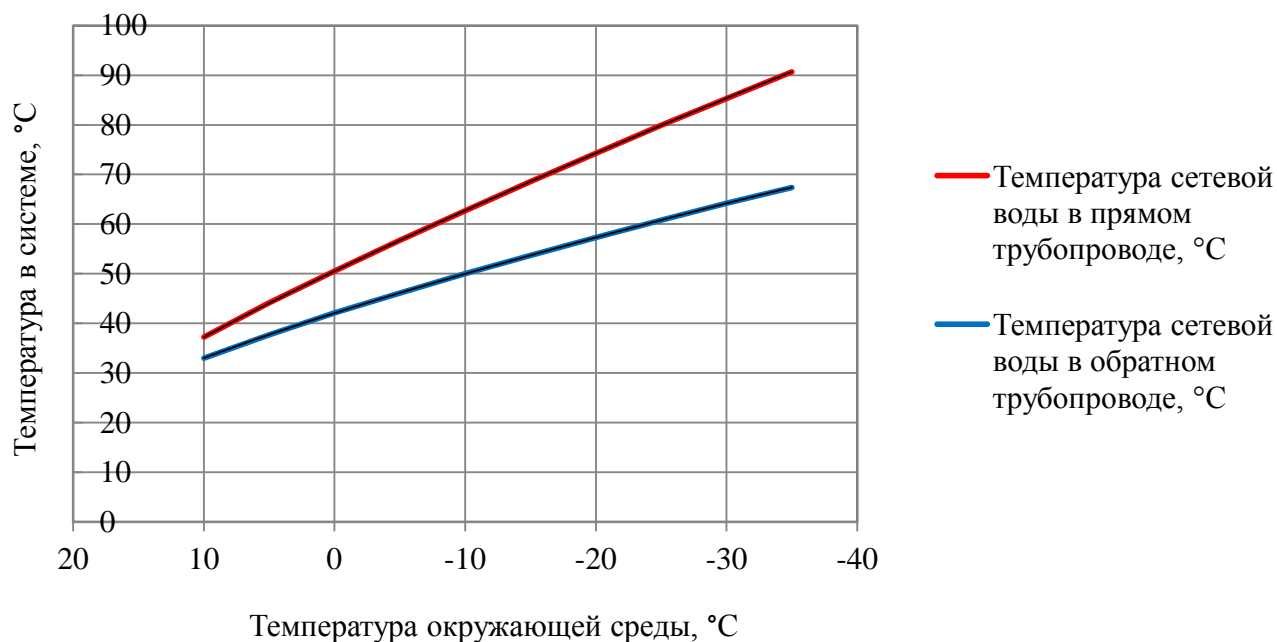
Рисунок 2.3 – График изменения температур теплоносителя
