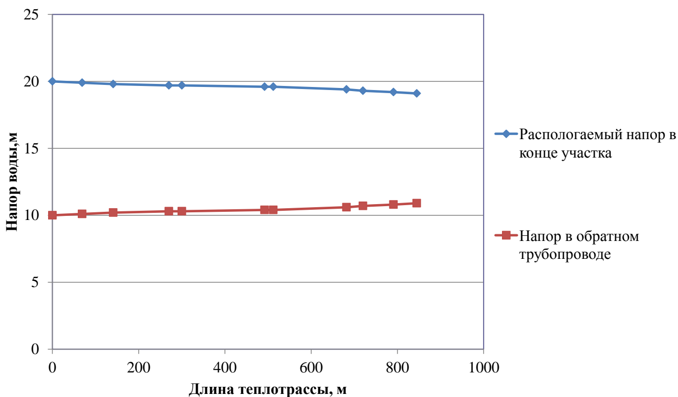
Рисунок 2.4 – Пьезометрический график тепловой сети котельной №2
